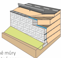
Stabilizácia a separácia zemín
